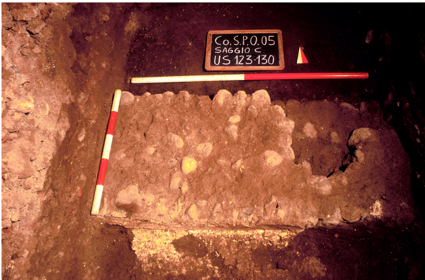
Fig. 4. Saggio C: muro di probabile età altomedievale.
